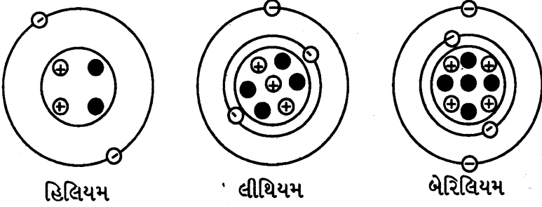
આકૃતિ - ૩ હિલિયમ, લીથિયમ, બેરિલિયમ
